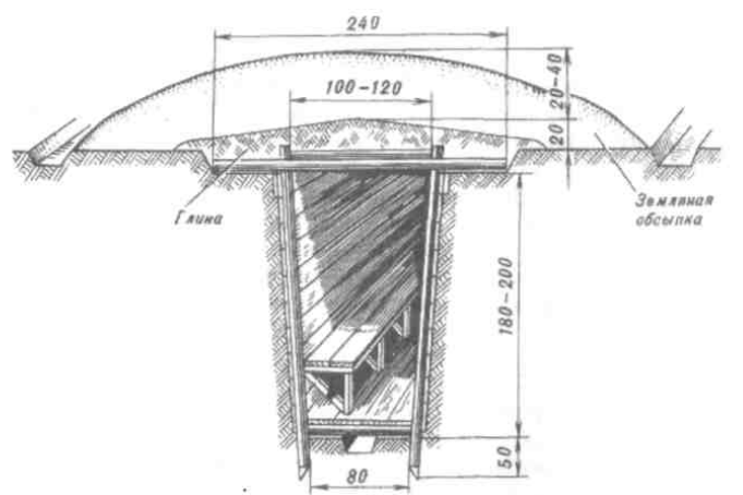
Рис.11. Перекрытая щель
