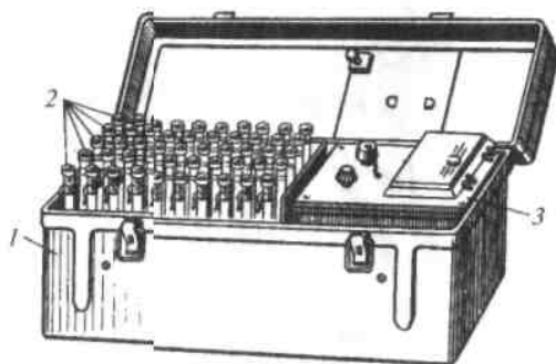
Рис. 2. Комплект индивидуальных дозиметров ДП-22В: 1 — укладочный ящик; 2 - дозиметры ДКП-50А; 3 - зарядное устройство ЗД-5
