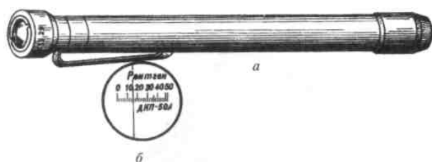
Рис. 3. Дозиметр ДКП-50А: а — общий вид; б—шкала
