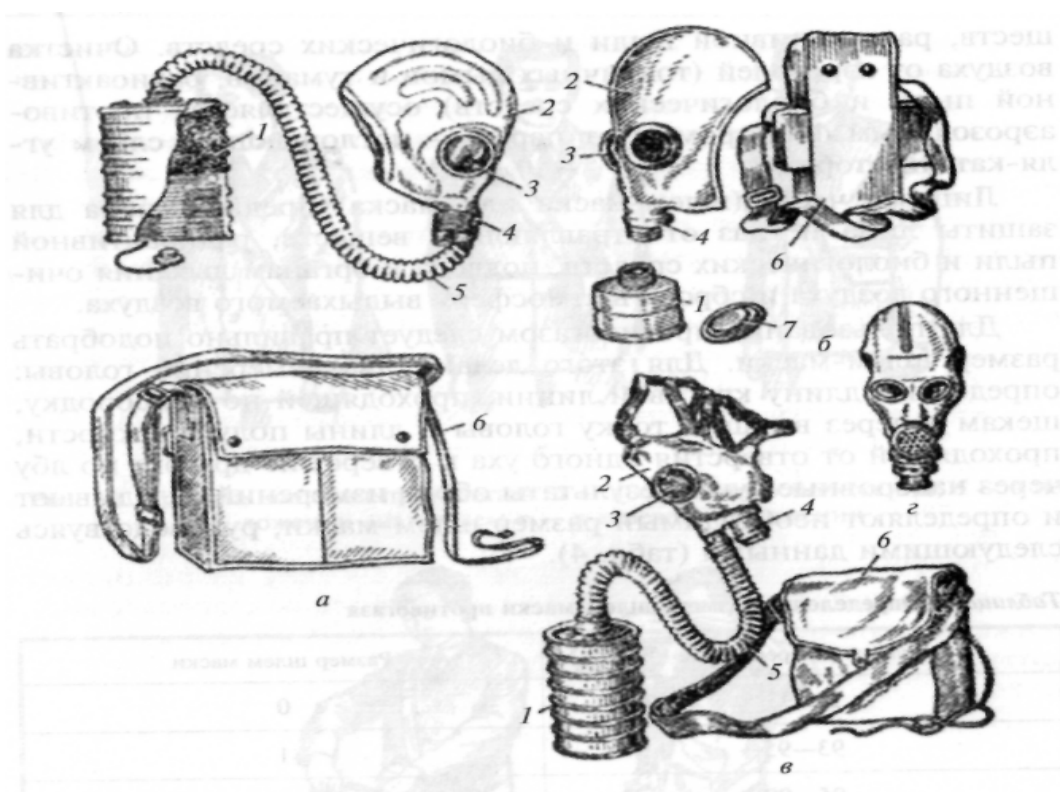
Рис. 1. Фильтрующие противогазы: а — общевойсковой противогаз; б — противогаз ГП-5; в — противогаз ГП-4у; г — шлем-маска с мембранной коробкой, входящая в комплект противогаза общевойскового и ГП-5М; / — фильтрующе-поглощающая коробка; 2 — лицевая часть (у противогаза общевойскового и ГП-5 — шлем-маска; у противогаза ГП-4у — маска); 3 — очковый узел; 4 — клапанная коробка; 5 — соединительная трубка; 6 — сумка для противогаза; 7 — коробка с незапотеваящими пленками
