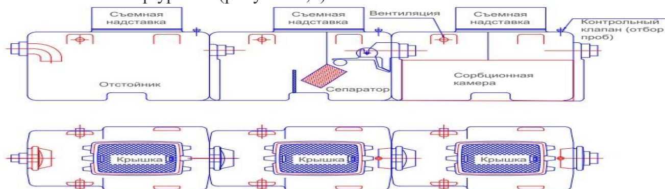
Рис 1. Нефтеуловитель
